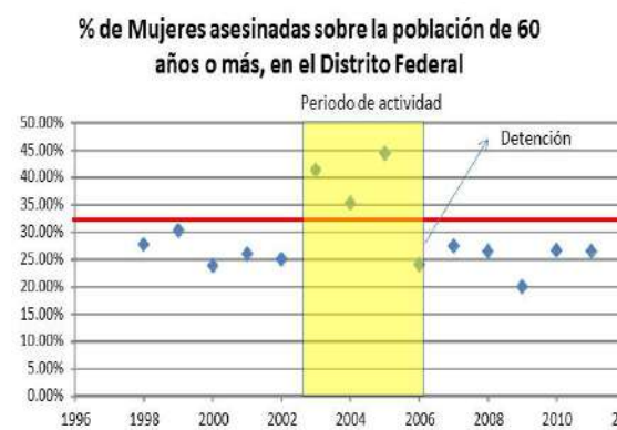
Gráfica 2. Aumento de ancianas asesinadas durante el periodo de actividad de Juana Barraza
